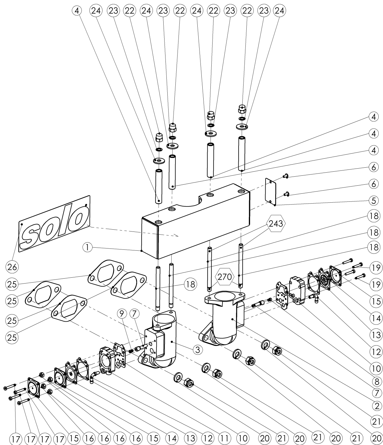
Bild 4 Vergaseranlage-DG-LS-2350-Walbro
