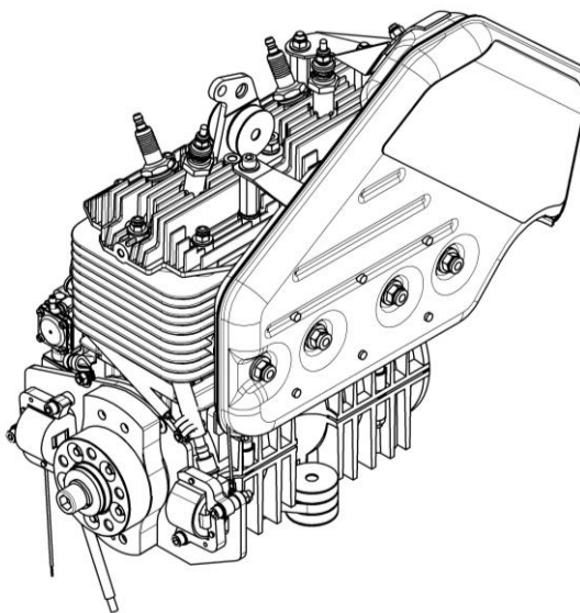
Flugmotor 2350 - LAK-Hedlitz-Zylinderköpfe
