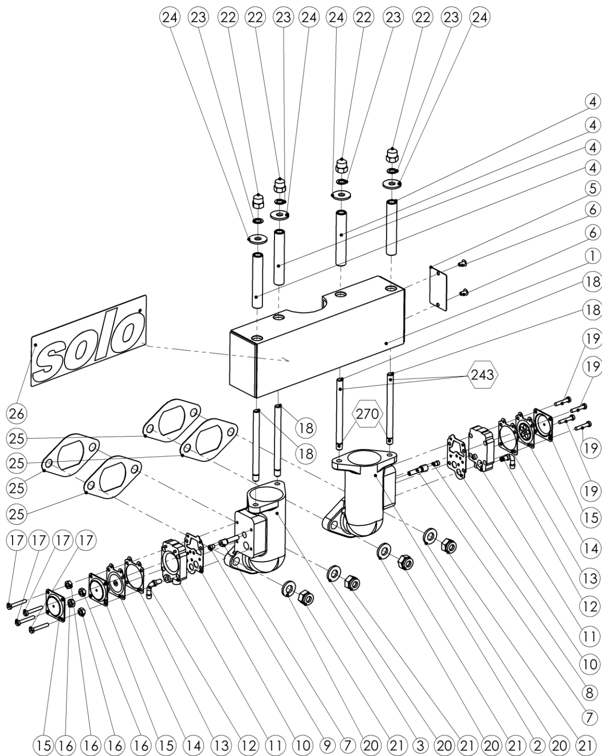
Bild 4 Vergaseranlage-LAK-2350-Walbro
