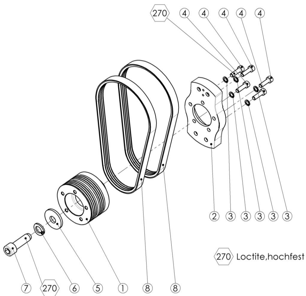
Bild 8 Abtriebswelle 2350D
