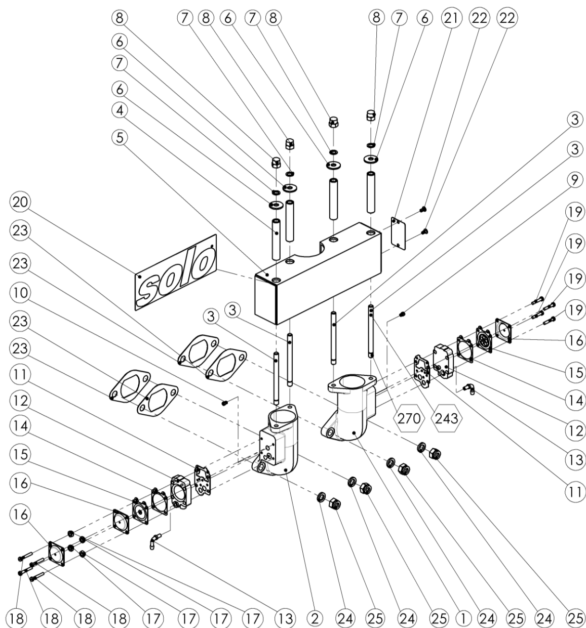
Bild 4 Vergaseranlage 2350D
