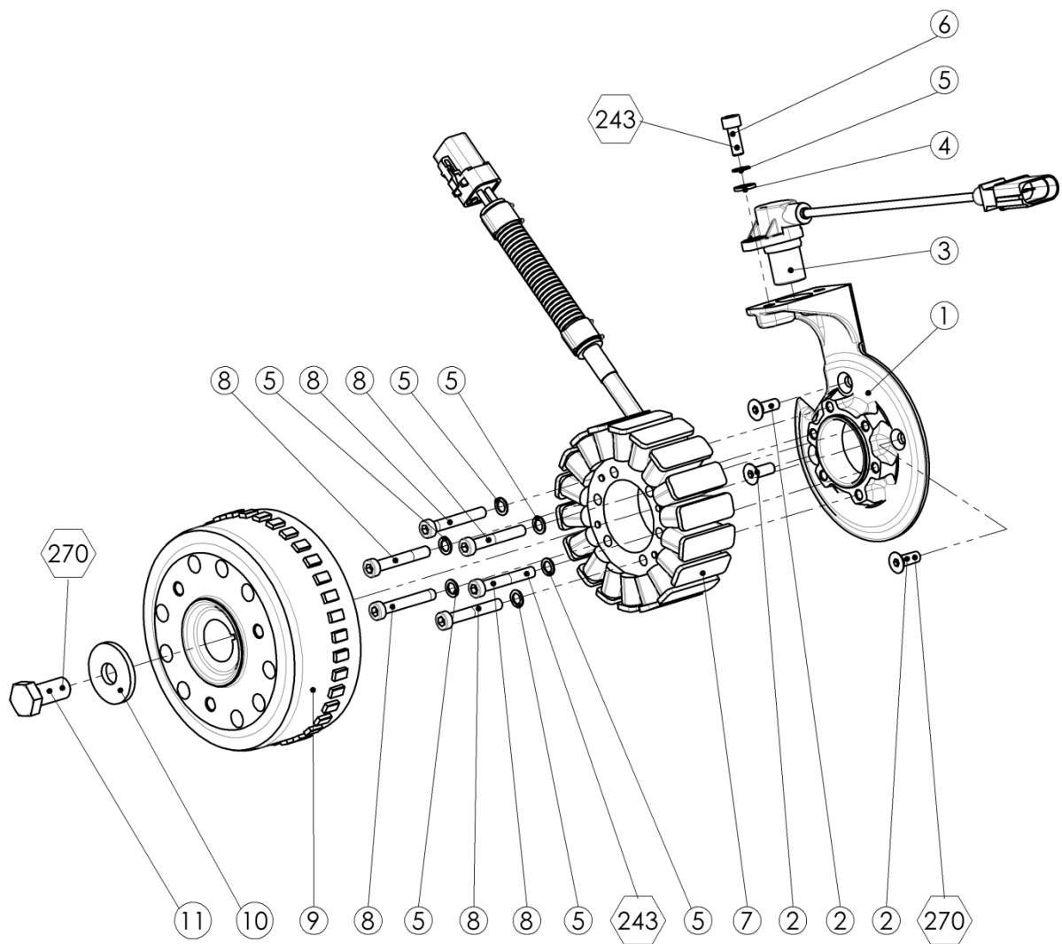
Bild 4 Zündung 2625-02i
