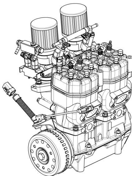
Bild 0 Flugmotor-2625-02-Binder
